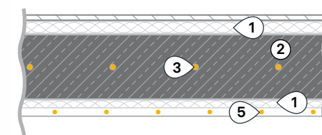
Integrierter Deckenspeicher* mit Klimadecke
