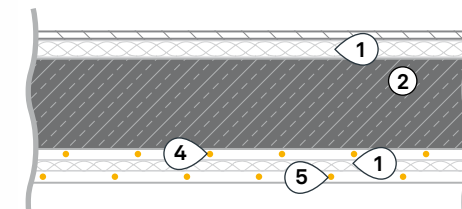
Nachträglich montierter Deckenspeicher* mit Klimadecke
